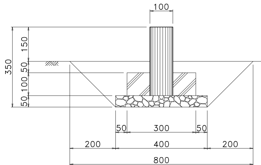
標準基礎図
