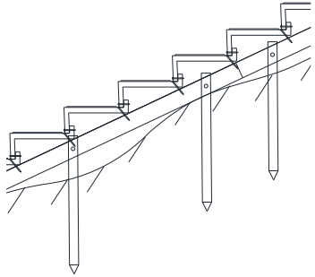
①柔らかな地面施工
