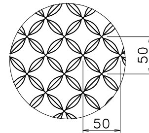
横木角材表面滑り止め形状
