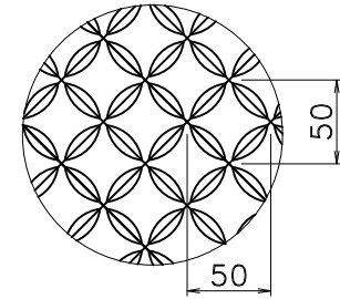
横木角材表面滑り止め形状
