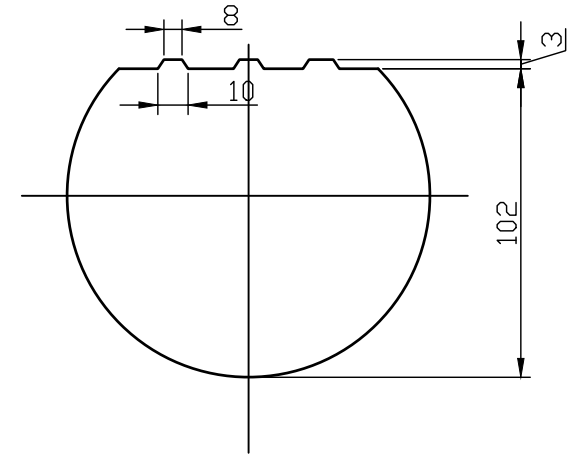
滑り止め処理詳細
