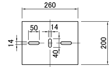
つなぎ板 ATGE-26長穴加工 詳細図 S=1:10
