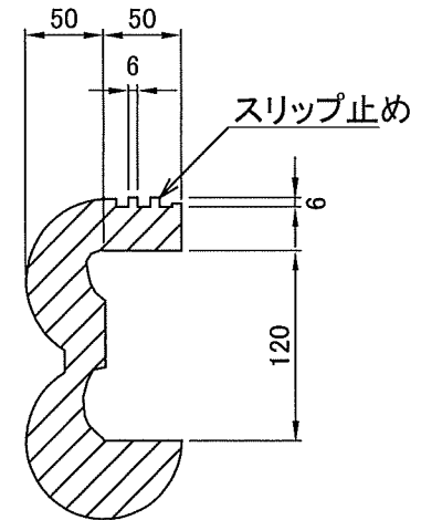
A-A断面 S=1:5
