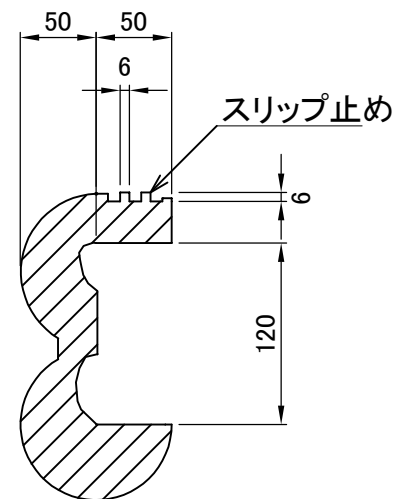
A-A断面 S=1:5
