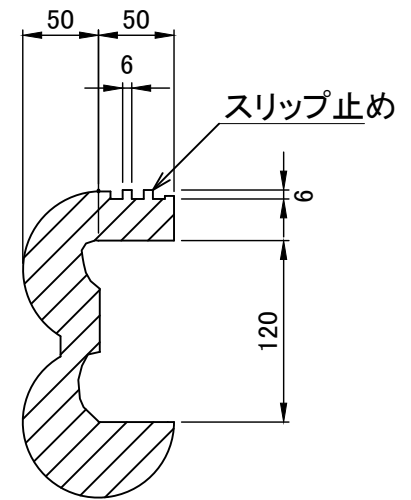
A-A断面 S=1:5
