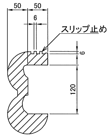
A-A断面 S=1:5
