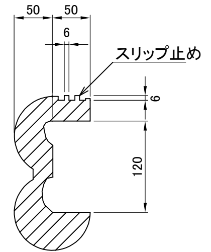
A-A断面 S=1:5
