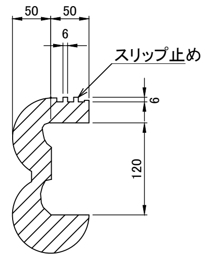
A-A断面 S=1:5
