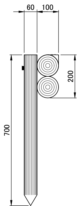
A-A断面 S=1:5
