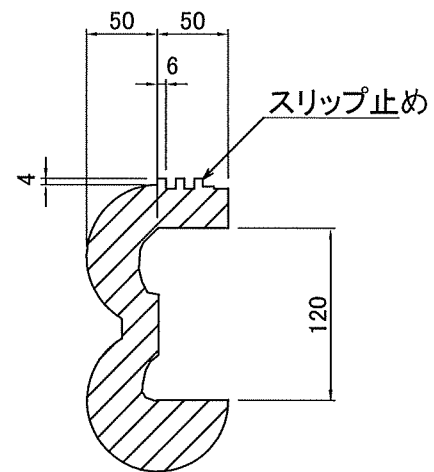
A-A断面 S=1:5
