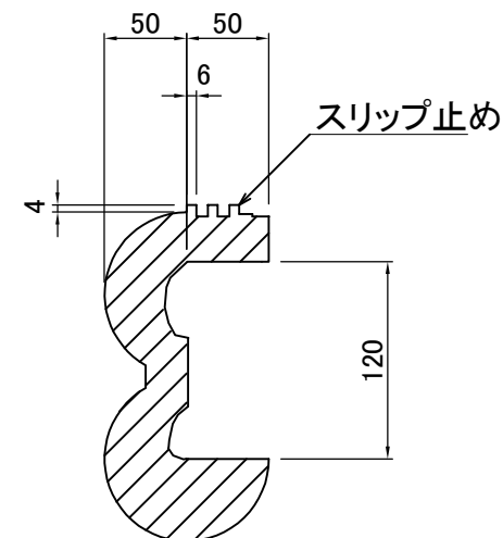
A-A断面 S=1:5
