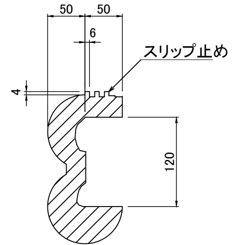
A-A断面 S=1:5
