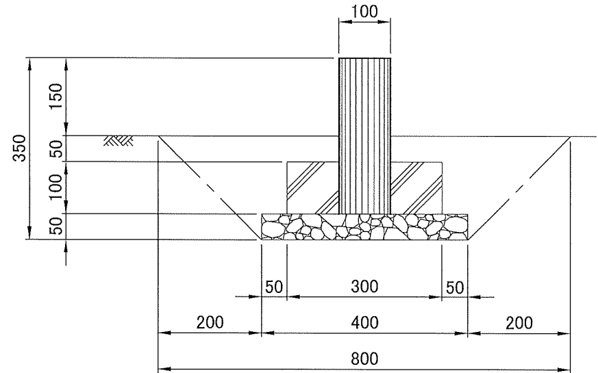
標準基礎図
