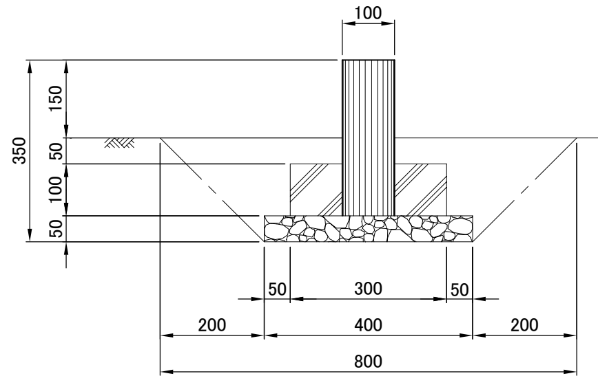
標準基礎図
