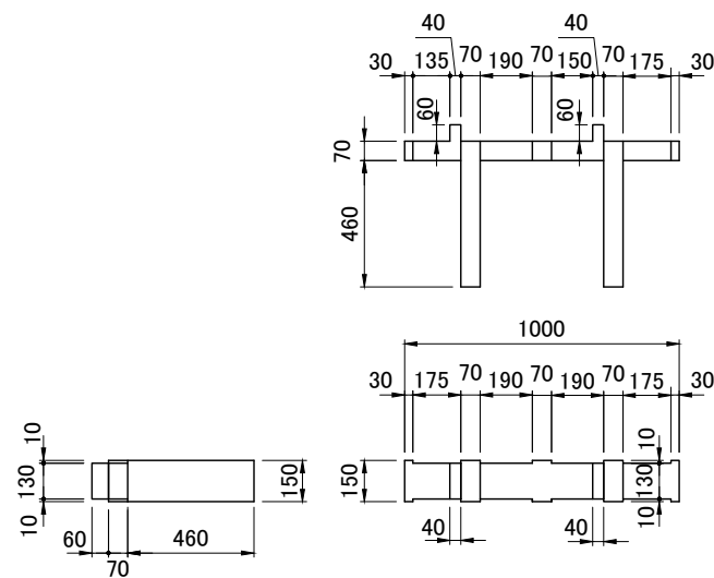
根太材 C
