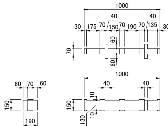
根太材 B
