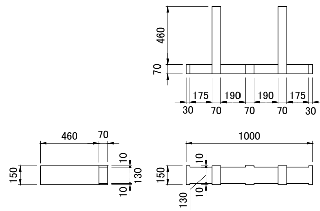
根太材 A
