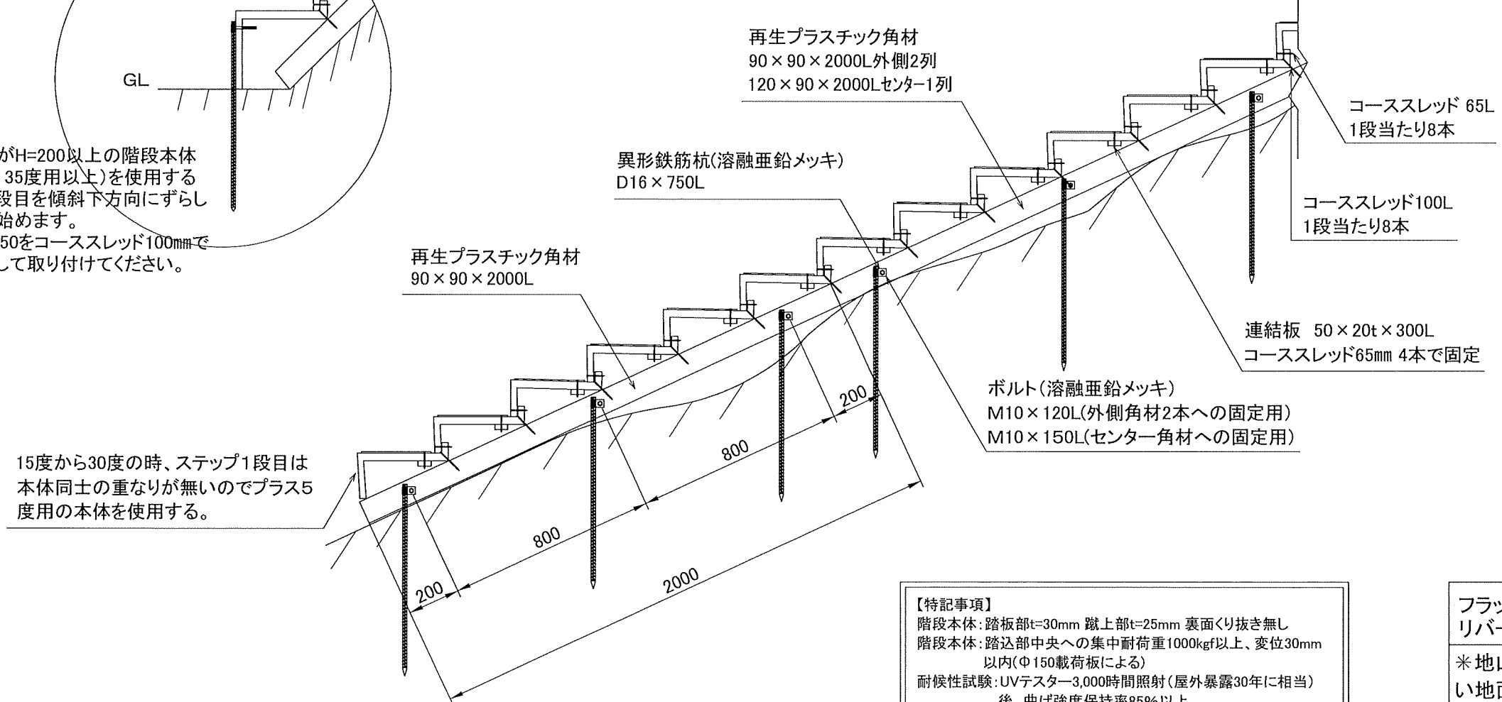
側面図 S=1:20
