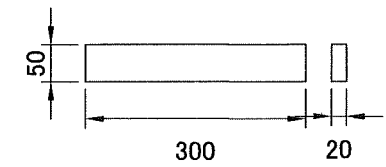
連結板 50×20t×300L
