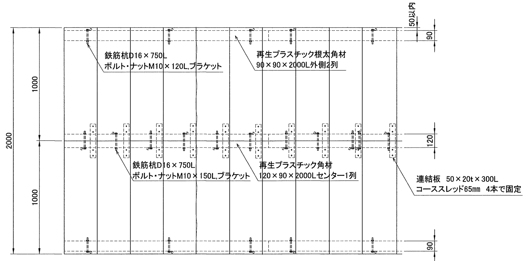
平面図 S=1:20
