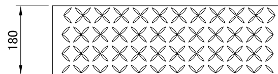
階段踏み板180×100×600
