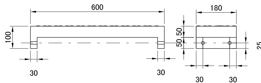
階段踏み板180×100×600
