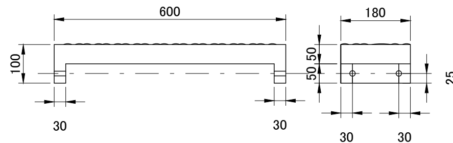
階段踏み板180×100×600
