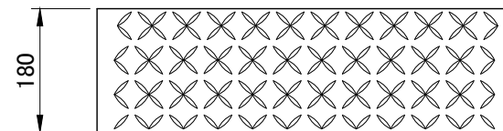
階段踏み板180×100×600
