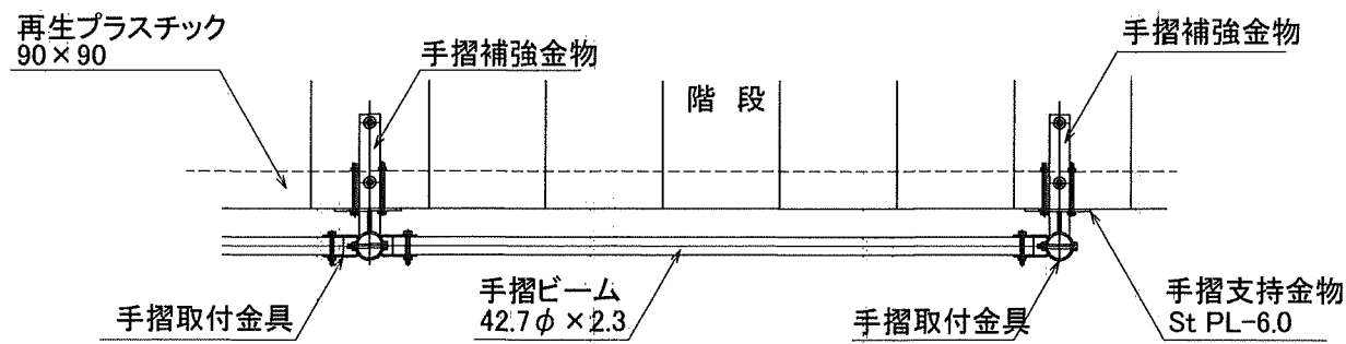
平面図 S=1:20
