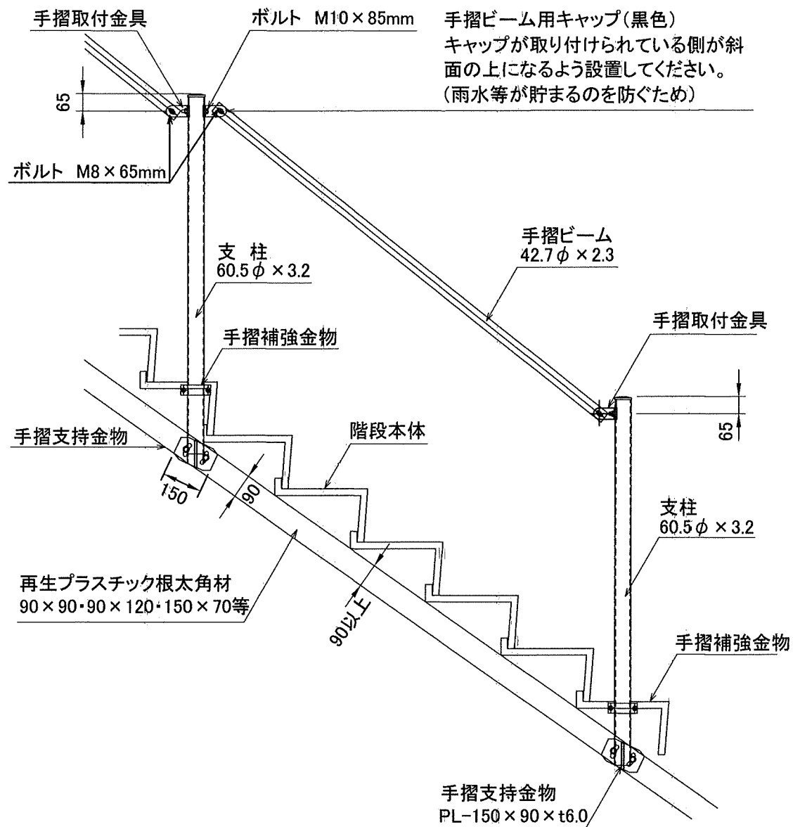
側面図 S=1:20
