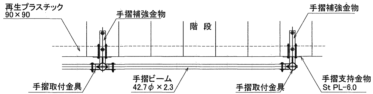
平面図 S=1:20
