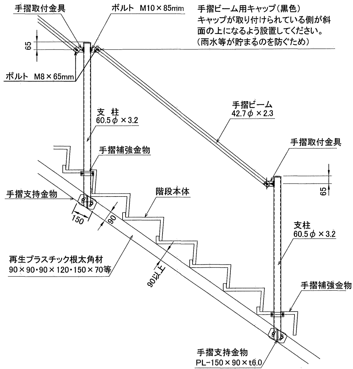
側面図 S=1:20
