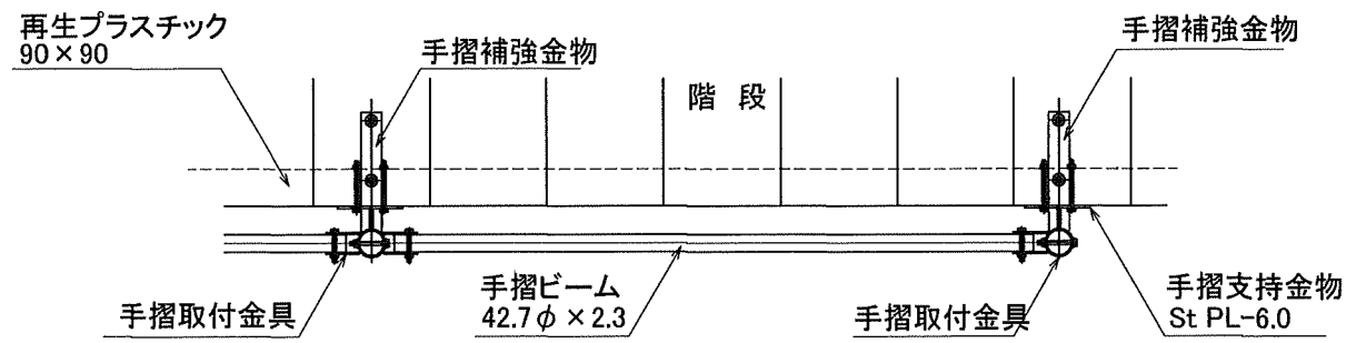
平面図 S=1:20
