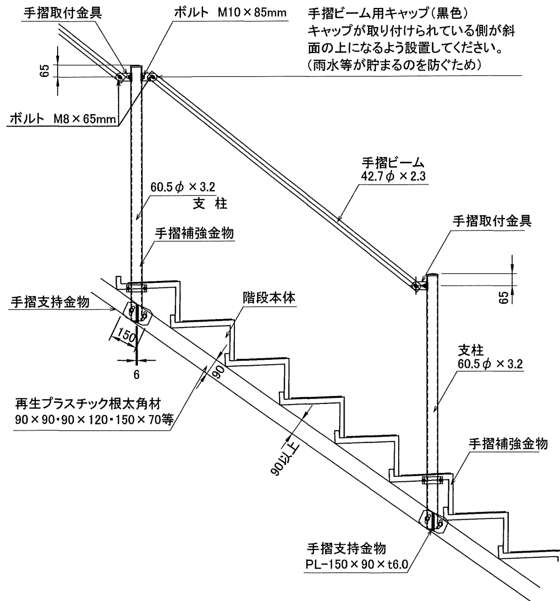
側面図 S=1:20
