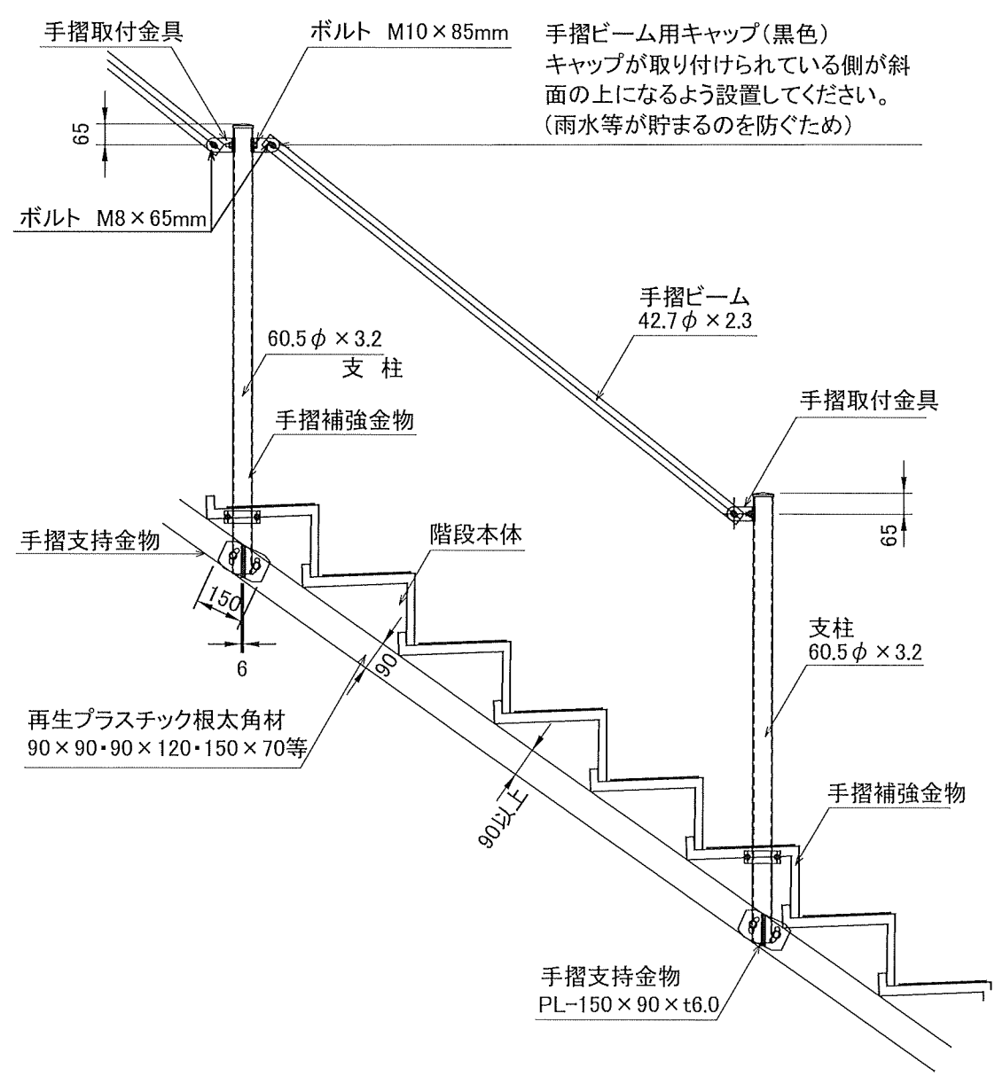
側面図 S=1:20
