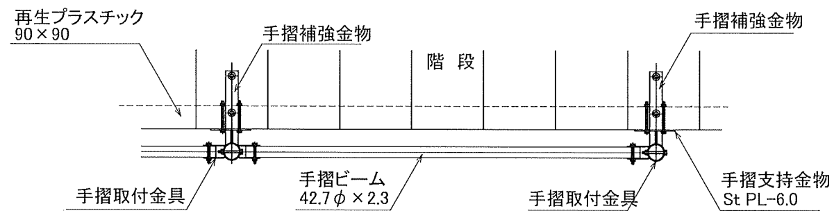
平面図 S=1:20
