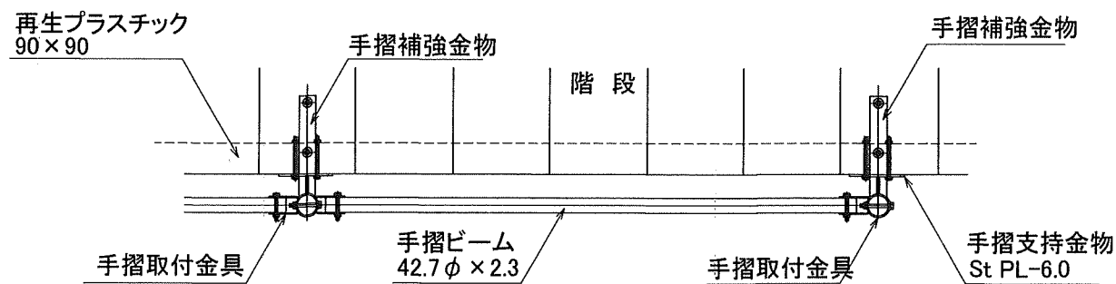
平面図 S=1:20
