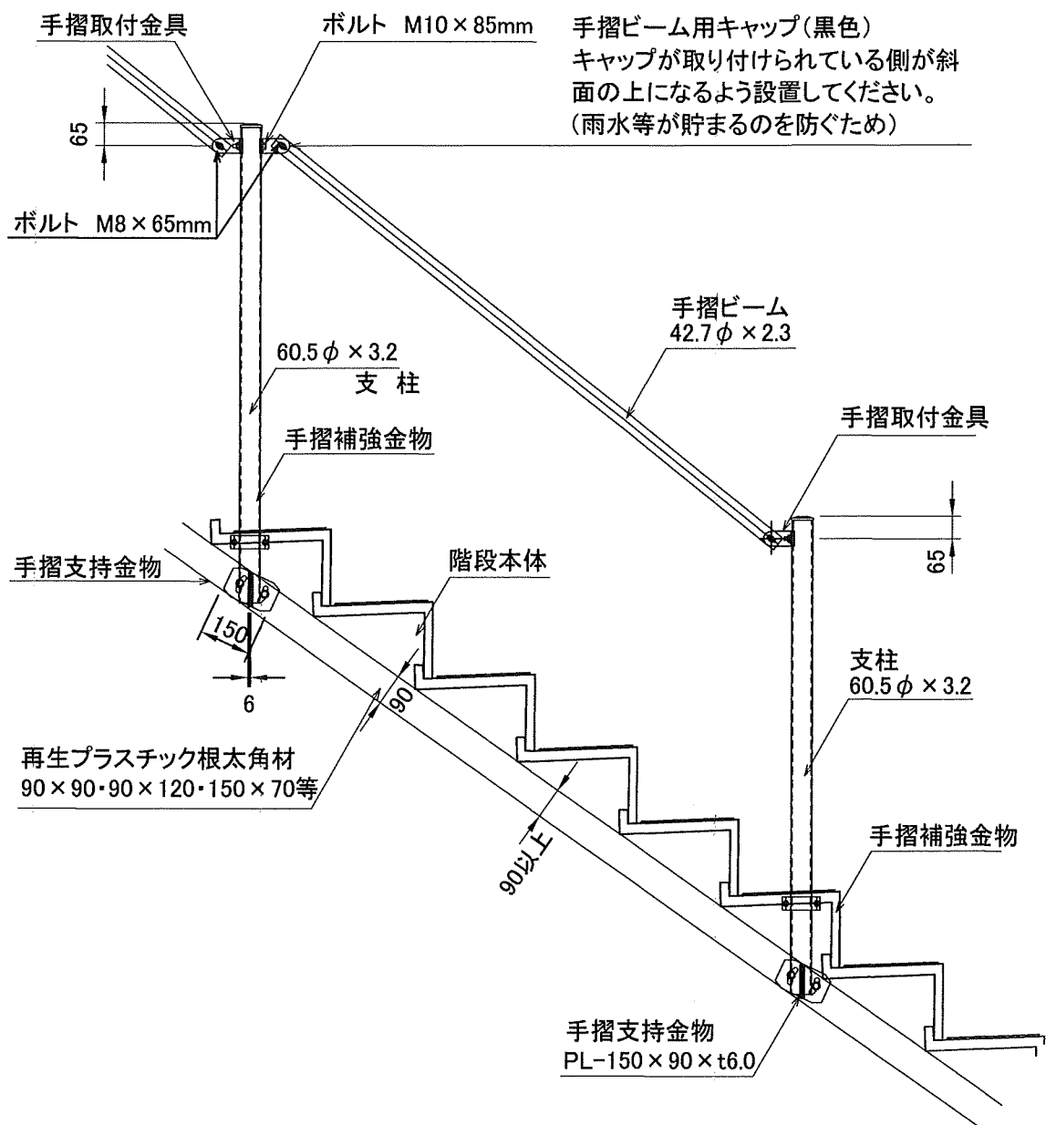
側面図 S=1:20
