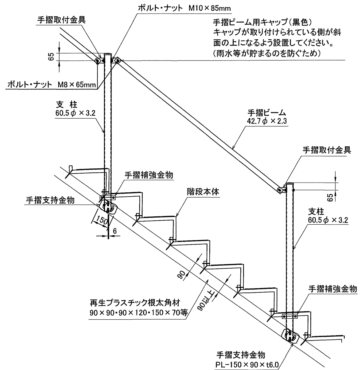
側面図 S=1:20
