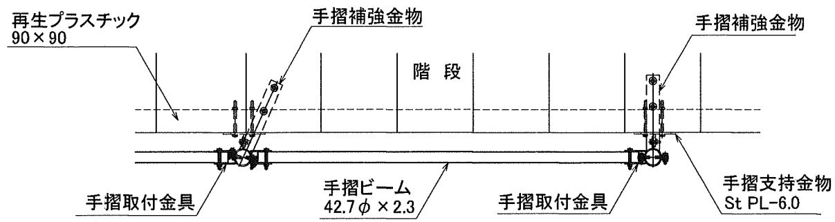
平面図 S=1:20
