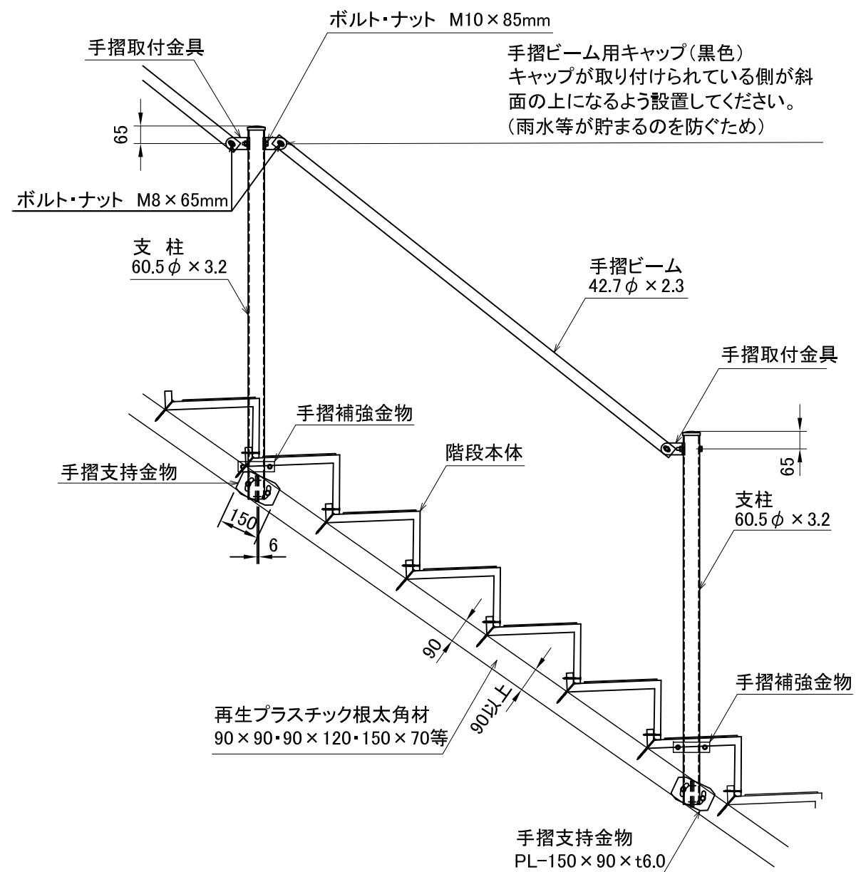
側面図 S=1:20
