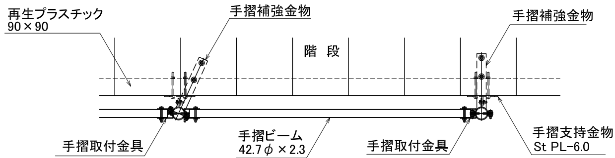
平面図 S=1:20
