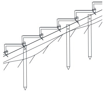
①柔らかな地面施工
