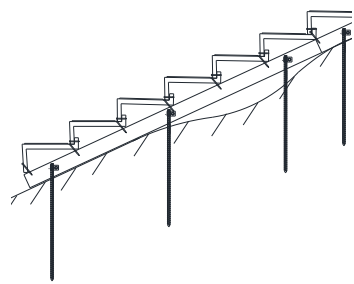
②硬い地山施工
